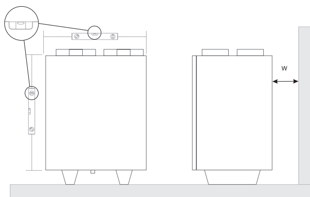
Figure 5.5.1 Positions horizontales de montage au sol (l = 400 mm)
