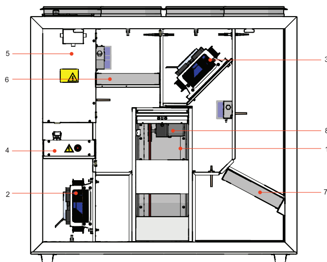
1 - Échangeur de chaleur rotatif; 2 - Ventilateur de soufflage; 3 - Ventilateur d'extraction; 4 - Batterie de chauffage électrique; 5 - Carte contrôleur ; 6 - Filtre pour air repris (panel); 7 - Filtre pour air soufflé (panel); 8 - Moteur à rotor.
