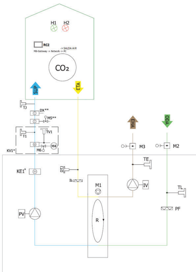
Figure 5.4.1 * KE1 - uniquement en version électrique ; * KV1 - utilisé dans la version à eau ; ** Possibilité de contrôler.
