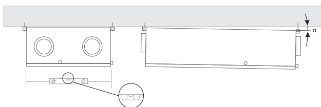
Потолочные крепления ( \alpha > 1^\circ )
