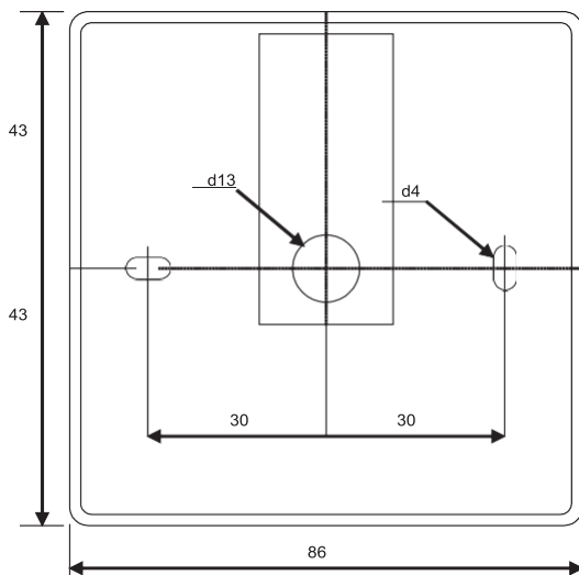
Чертеж сборки
