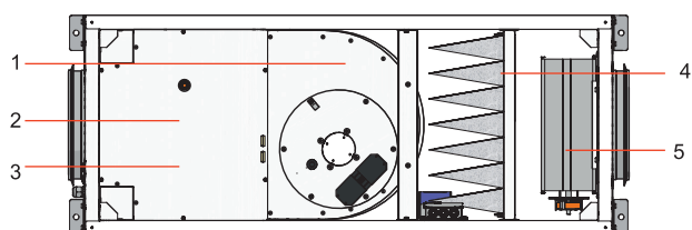
Рисунок 4.6.1 AmberAir Compact VEKA INT 400-700 EKO
