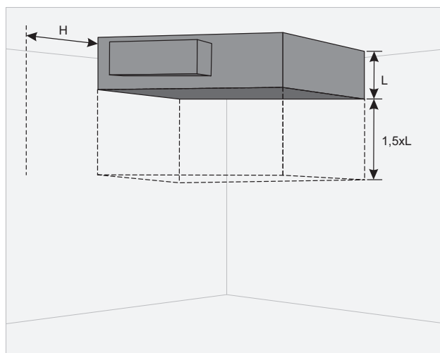
Рисунок 5.5.1.1 Мин. расстояние до открытия двери - 1,5 \times L ; Мин. расстояние до открытия двери блока управления - H > 400 мм.
