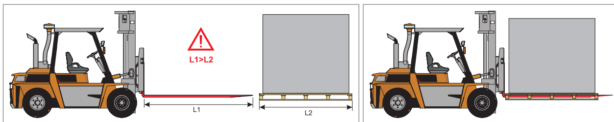
Рисунок 5.2.1 Подъем на вилочном погрузчике.
