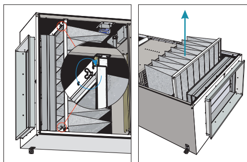
Рисунок 6.4.1 AmberAir Compact VEKA INT EKO
