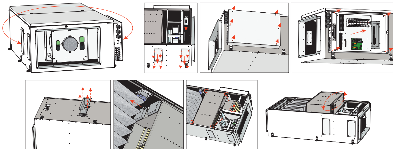
Рисунок 5.5.3 AmberAir Compact VEKA INT 3000-4000 ЕКО изменение стороны обслуживания
