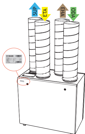
Abbildung 2.3 Platzierung Typenschild und Luftkanalanschluss (rechte Seite)
