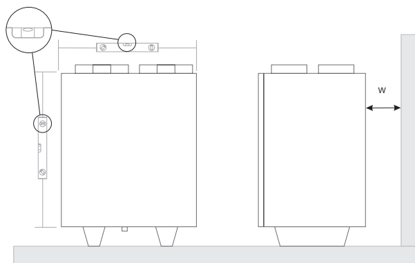
Abbildung 5.5.1 Montageposition: Horizontal Boden (W=400mm)
