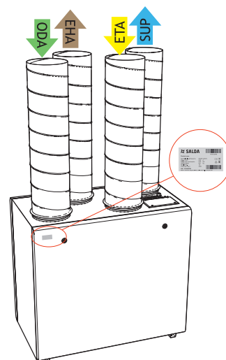
Abbildung 2.4 Platzierung Typenschild und Luftkanalanschluss (linke Seite)
