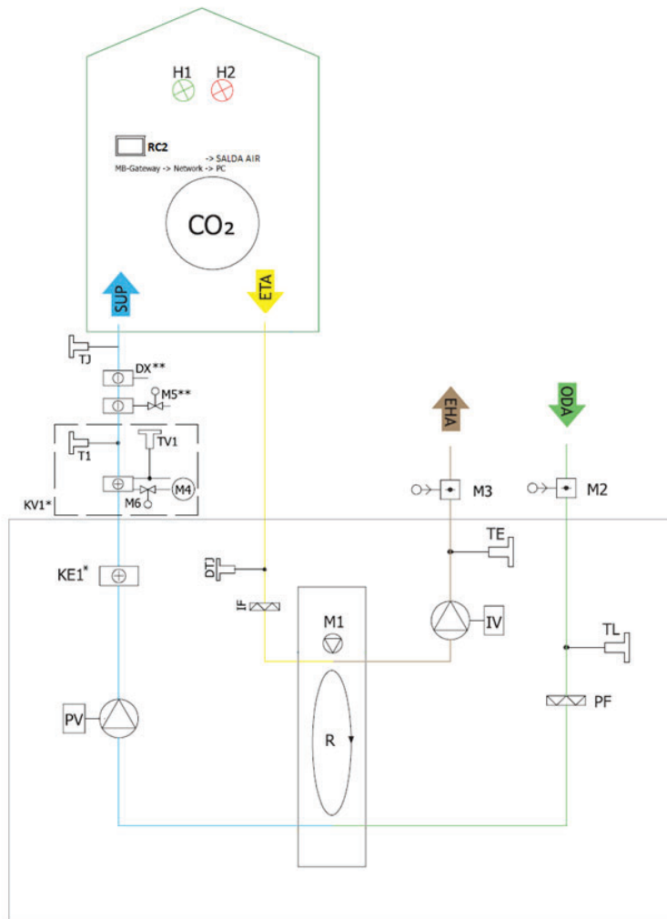
Abbildung 5.4.1 *KE1- nur Elektroversion; *KV1 - in Wasserversion verwendet; **Steuerung möglich.
