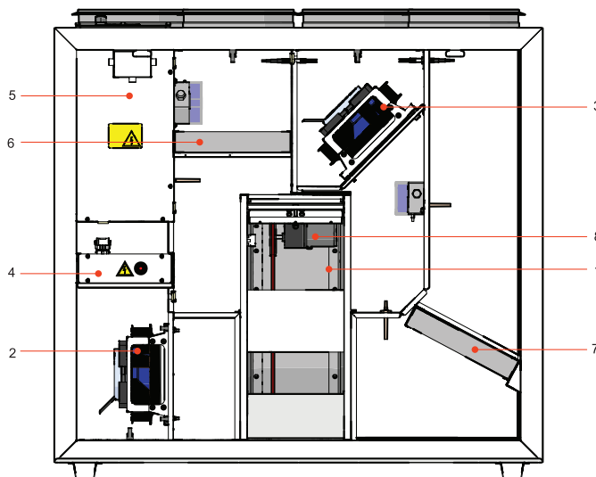
1 - Rotorwärmetauscher; 2 - Zuluftventilator; 3 - Abluftventilator; 4 - Elektroheizregister; 5 - Steuerungsplatine; 6 - Abluftfilter (Panelfilter); 7 - Zuluftfilter (Panelfilter); 8 - Rotorantrieb.
