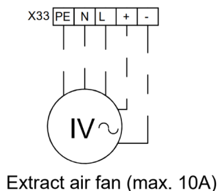
Rys. 8.5.1 AmberAir Compact VEKA INT EKO 400-1000
