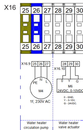
Rys. 8.4.2 AmberAir Compact VEKA INT EKO 3000-4000 W
