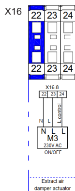
Rys. 8.2.2 AmberAir Compact VEKA INT EKO 3000-4000 W
