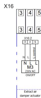
Rys. 8.2.3 AmberAir Compact VEKA INT EKO 2000
