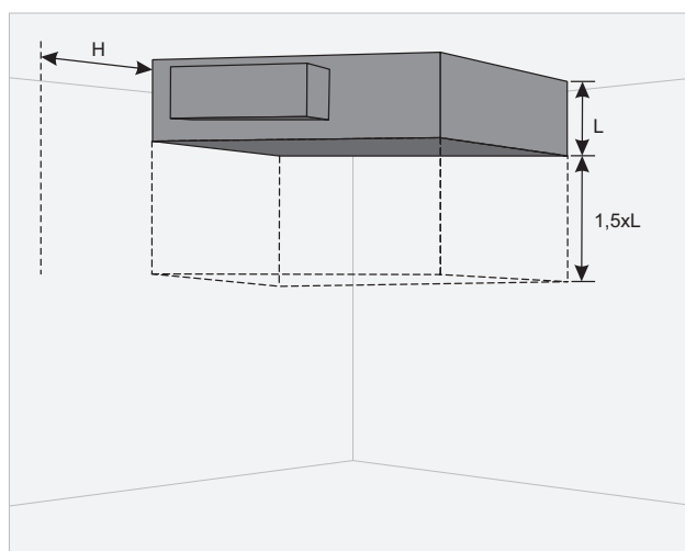
Rys. 5.5.1.1 Min. odległość na otwarcie drzwi – 1,5xL ; Min. odległość na otwarcie drzwi panelu sterowania – H > 400 \text{ mm} .
