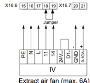
Rys. 8.5.3 AmberAir Compact VEKA INT EKO 3000-4000
