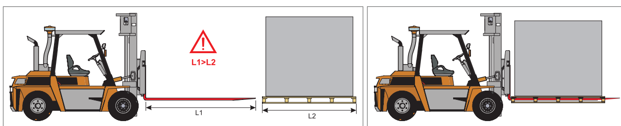
Rys. 5.2.1 Podnoszenie wózkiem widłowym
