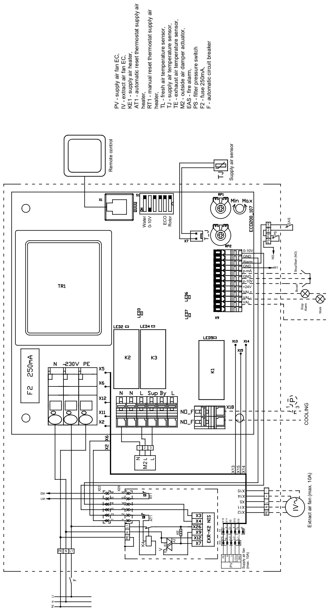
Rys. 8.7.4 AmberAir Compact VEKA INT EKO 1000-2.4
