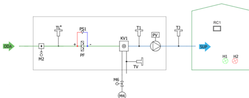
Pav. 5.4.1 AmberAir Compact VEKA INT W EKO (* AmberAir Compact VEKA 1000-2000 įrenginiams TL yra išorėje, kairėje nuo M2)
