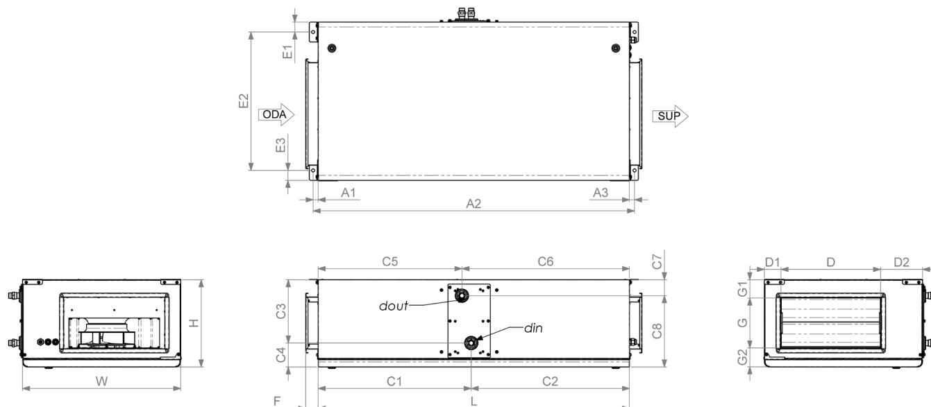
Pav. 4.2.1 AmberAir Compact VEKA INT 400-700 EKO
