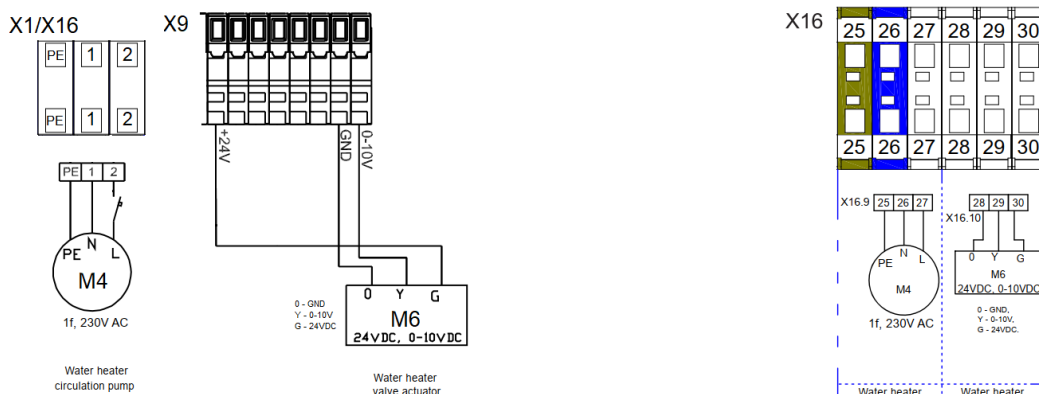
Pav. 8.4.1 AmberAir Compact VEKA INT EKO 1000-2000 W
