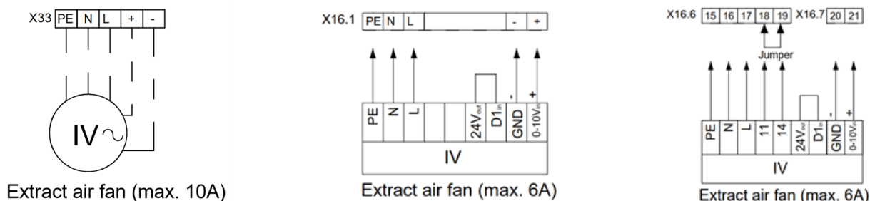
Pav. 8.5.1 AmberAir Compact VEKA INT EKO 400-1000
