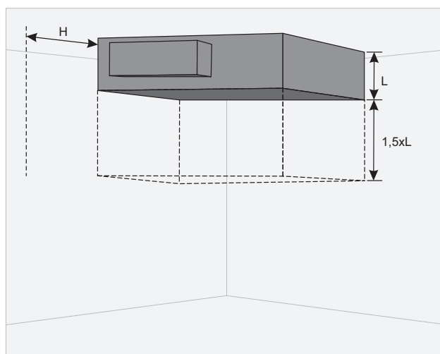
Pav. 5.5.1.1 Minimalus atstumas durims atidaryti - 1,5xL ; Minimalus atstumas atidaryti automatikos dėžės dangtį - H > 400 \text{ mm} .
