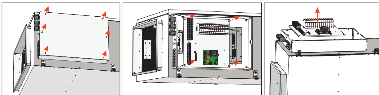
Pav. 6.7.2 AmberAir Compact VEKA INT 3000-4000 EKO
