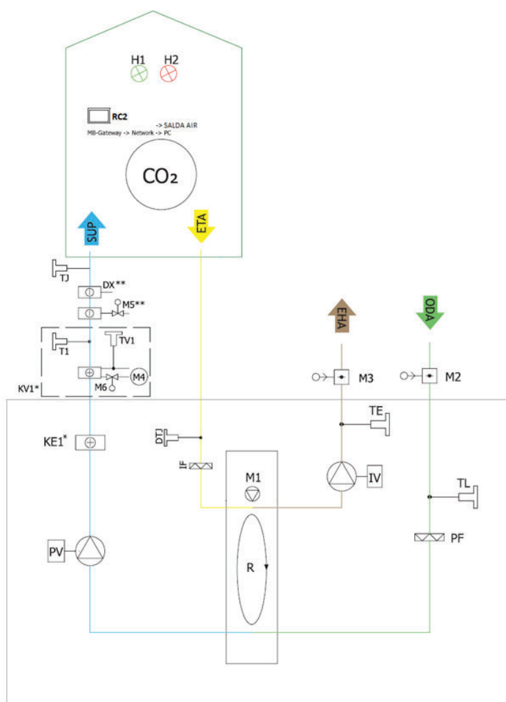
Rys. 5.4.1. * KE1 – tylko w wersji z nagrzewnicą elektryczną; * KV1 – stosowane w wersji z nagrzewnicą wodną; ** Możliwość sterowania.
