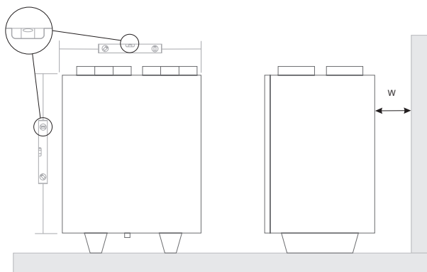
Rys. 5.5.1. Położenie do montażu poziomego na podłodze (szer. = 400 mm)
