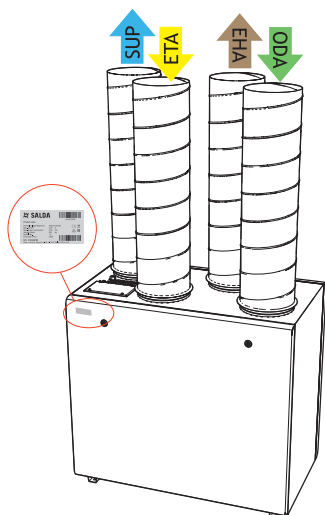
Rys. 2.3. Umieszczenie etykiety technicznej i oznaczenie króćców powietrza (prawa strona)
