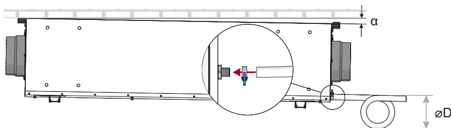
Рисунок 5.5.2.2 Монтаж дренажной системы ( \varnothing D=150 мм) (только для установок с конденсирующим теплообменником)
