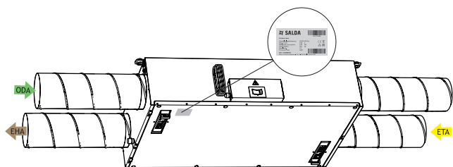
Рисунок 2.3 Smarty 2X P S300 Расположение технической этикетки и индикация воздушного канала
