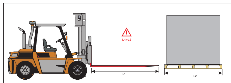
Рисунок 5.2.3 Подъем на вилочном погрузчике.
