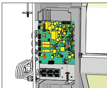
Рисунок 6.8.4 Smarty 3/4X P S300
