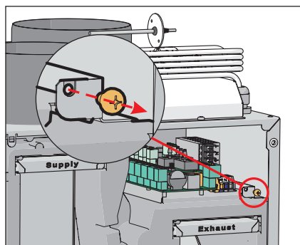
Рисунок 6.8.5 Smarty 2/3/4X V 1.1/1.2
