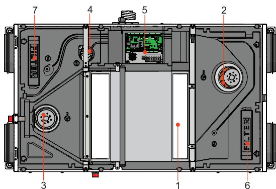
Рисунок 4.6.2 Smarty 2X P 1.1/1.2
