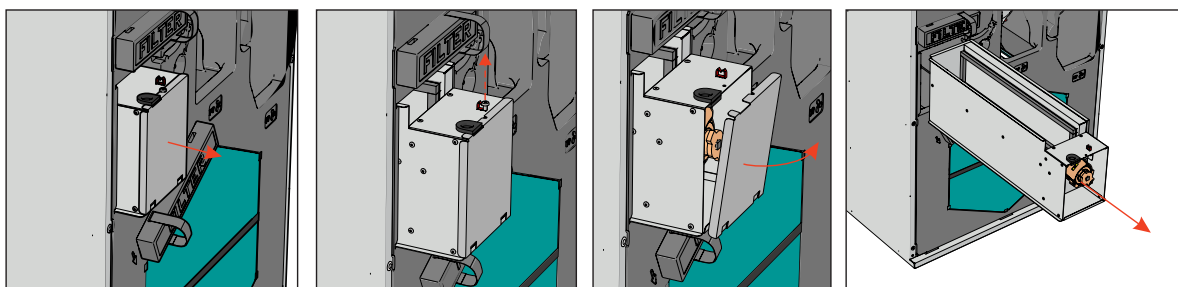
Рисунок 6.7.8 Smarty 3X V / 4X V S300
