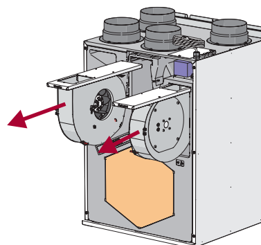
Рисунок 6.6.10 Smarty 3X V / 4X V
