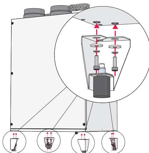
Рисунок 5.5.3.1 Крепление к полу (требуется дополнительное оборудование)
