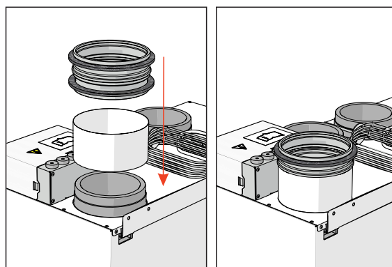
Рисунок 5.6.3 Подключение воздуховода для Smarty 2X V S300
