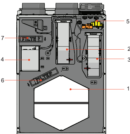
Рисунок 4.6.9 Smarty 3X V / 4X V S300
