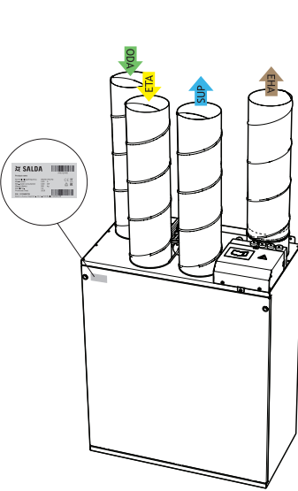
Рисунок 2.6 Smarty 2X V S300 Расположение технической этикетки и индикация воздушного канала
