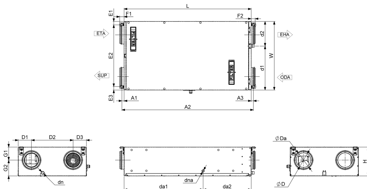
Рисунок 4.2.2 Smarty 2X P 1.1/1.2 1kW PH
