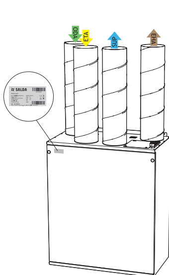
Рисунок 2.5 Smarty 2X V 1.1/1.2 Расположение технической этикетки и индикация воздушного канала
