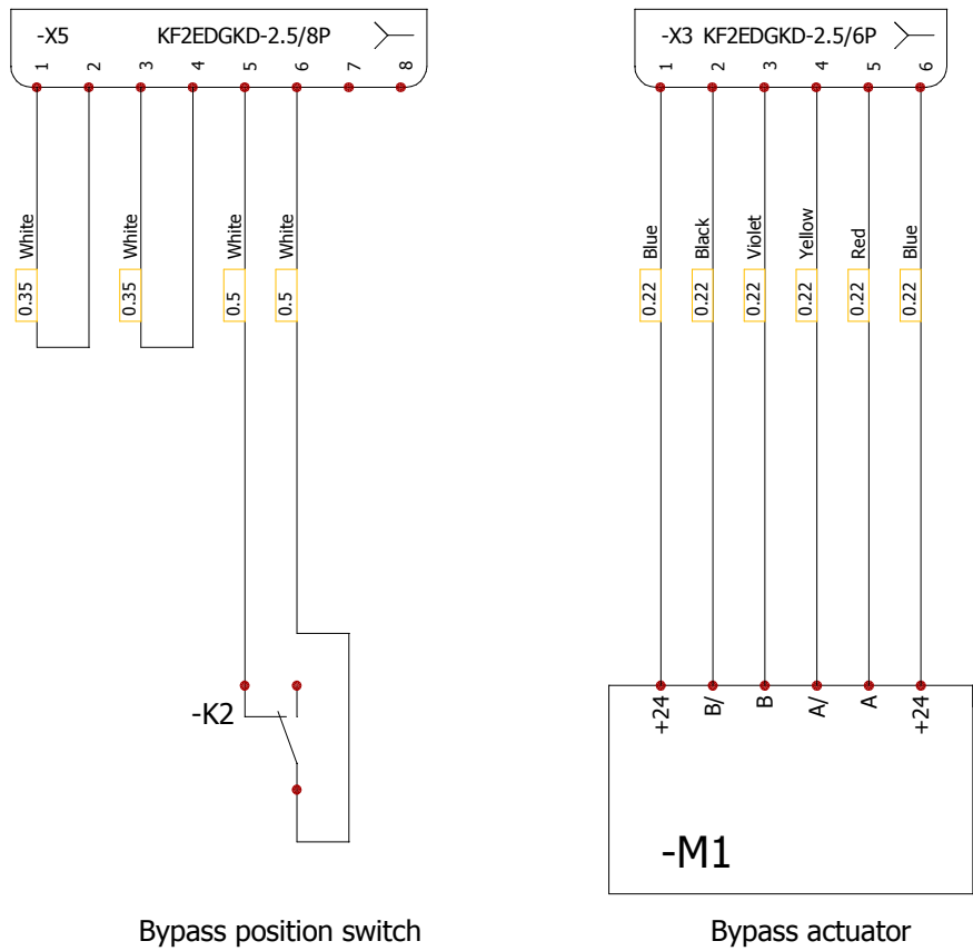
Рисунок 8.15.5 Схема подключения обхода (версия 1.1 / 1.2) (221.1055.0.1.0-PS)
