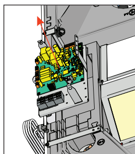
Рисунок 6.8.4 Smarty 3/4X P S300
