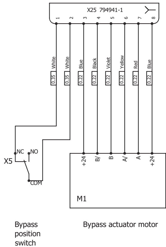
Рисунок 8.15.4 Обход (SMARTY ZP3X V-0k)
