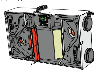
Рисунок 6.5.1 Smarty 2X P
