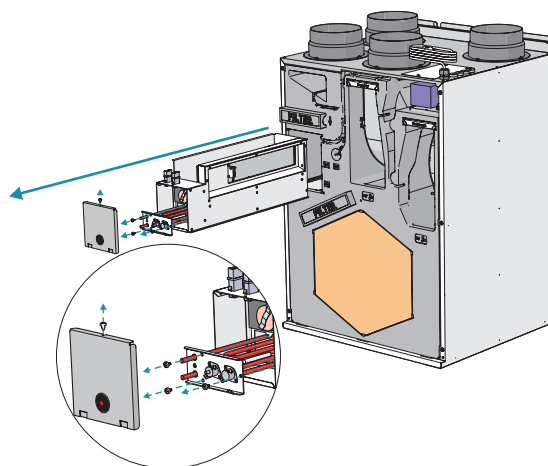
Рисунок 6.7.6 Smarty 3X V / 4X V F2 1.1/1.2 / Smarty 2X V 1.2 E 0.6kW PH
