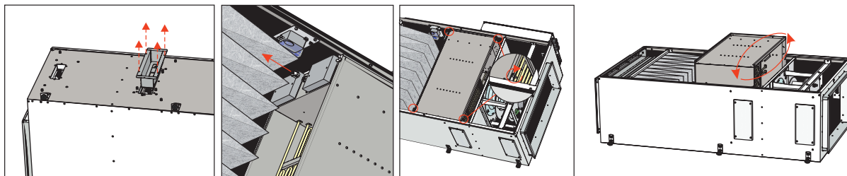
Abbildung 5.5.3 AmberAir Compact VEKA INT 3000-4000 EKO Wechsel der Wartungsseite
