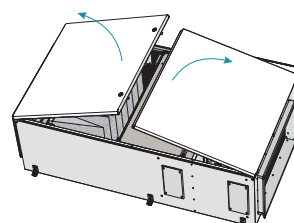
Abbildung 6.3.2 AmberAir Compact VEKA INT 3000-4000 EKO
