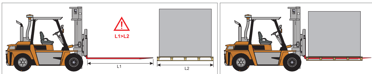
Abbildung 5.2.1 Heben mit Gabelstapler
