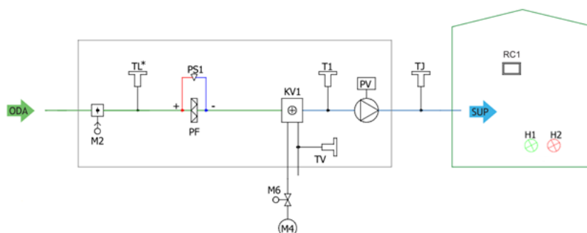
Abbildung 5.4.1 AmberAir Compact VEKA INT W EKO (*Für AmberAir Compact VEKA 1000-2000 Geräte befindet sich TL außerhalb des Geräts, links von M2)
