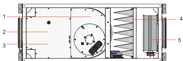
Abbildung 4.6.1 AmberAir Compact VEKA INT 400-700 EKO
