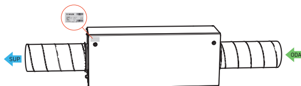
Abbildung 2.4 Platzierung Technischer Aufkleber und Luftkanalanschluss AmberAir Compact VEKA INT 400-700 E EKO
