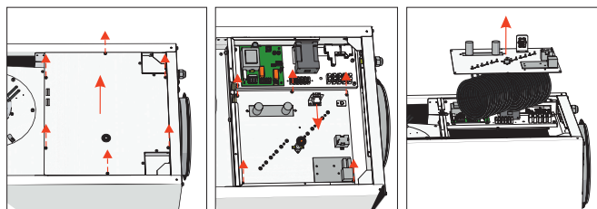
Abbildung 6.6.1 AmberAir Compact VEKA INT 400-700 E KO
