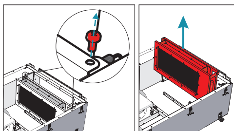
Abbildung 6.6.3 AmberAir Compact VEKA INT W KO
