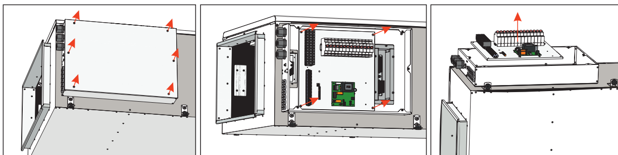
Abbildung 6.7.2 AmberAir Compact VEKA INT 3000-4000 EKO
