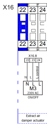
Abbildung 8.2.2 AmberAir Compact VEKA INT EKO 3000-4000 W
