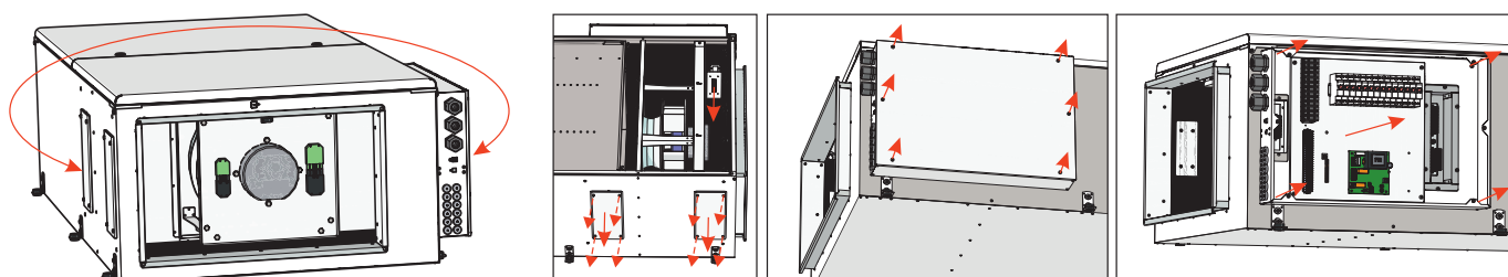
Abbildung 5.5.2 AmberAir Compact VEKA INT 400-700 EKO Wechsel der Wartungsseite
