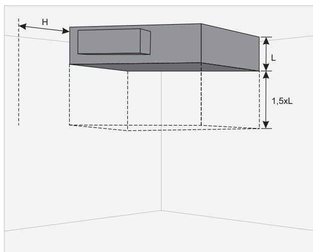
Abbildung 5.5.1.1 Min. Abstand für Türöffnung - 1,5xL ; Min. Abstand für Öffnung des Schaltkastens - H > 400 \text{ mm} .
