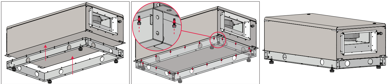
Abbildung 5.5.4.1 AmberAir Compact VEKA INT 1000-2000 EKO Bodenmontage (optionales Zubehör benötigt)
