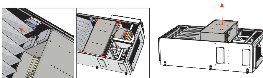
Abbildung 6.6.2 AmberAir Compact VEKA INT 1000-4000 E KO
