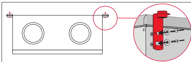
Abbildung 5.5.2.1 Deckenmontage
