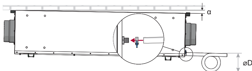
Figure 5.5.4. Installation du système de drainage ( \varnothing D=150 mm)
