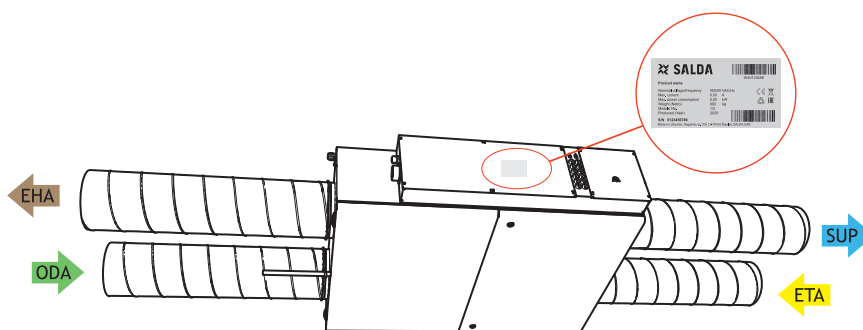
Figure. 2.3. Emplacement de l'étiquette signalétique et indication de raccordement des gaines
