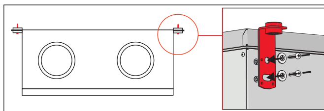
Figure 5.5.3. Positions d'installation au plafond
