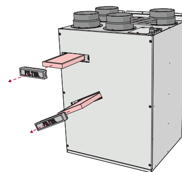
Afbeelding 6.4.3 Smarty 3X V / 4X V
