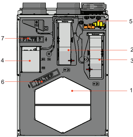
Afbeelding 4.6.9 Smarty 3X V / 4X V S300
