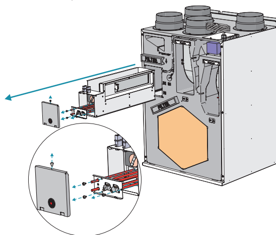
Afbeelding 6.7.6 Smarty 3X V / 4X V F2 1.1/1.2 / Smarty 2X V 1.2 E 0.6kW PH
