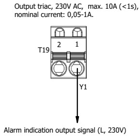
Afbeelding 8.13.1 Alarmindicatie-output verbinding
