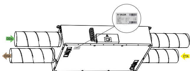
Afbeelding 2.3 Smarty 2X P S300 Kentekenplaatje en aanwijzing kanaalaansluiting
