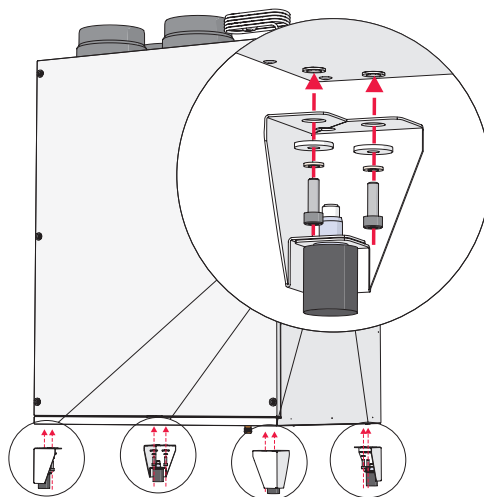
Afbeelding 5.5.3.1 vloermontage (accessoire in optie vereist)
