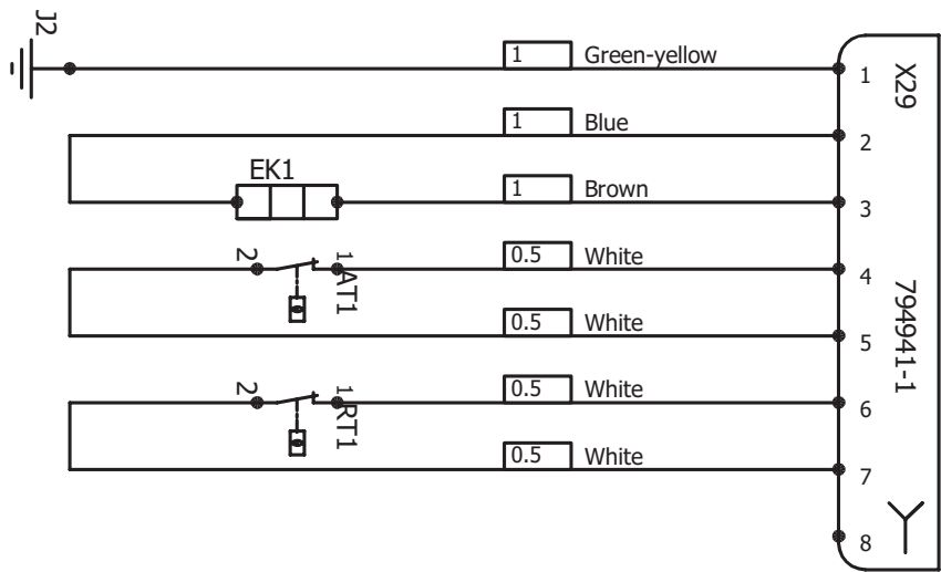
Afbeelding 8.15.7 Voorverwarmer (SP35)
