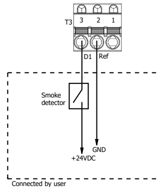
Afbeelding 8.3.1 Verbinding van rookdetector
