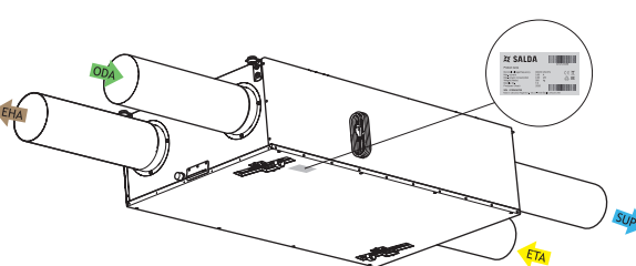
Afbeelding 2.4 Smarty 2X P 1.1 / 1.2, 3X P, 4X P Kentekenplaatje en aanwijzing kanaalaansluiting
