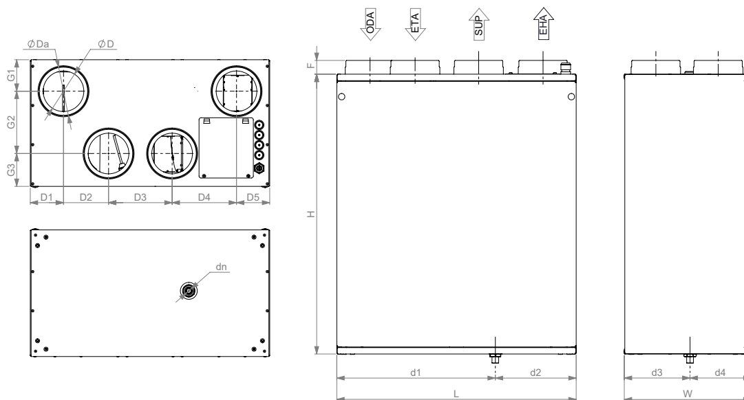
Afbeelding 4.2.4 Smarty 2X V 1.1/1.2
