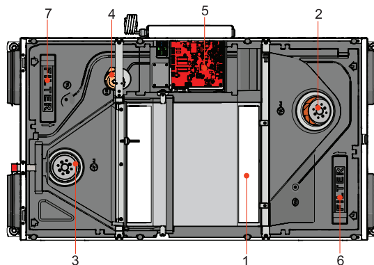
Afbeelding 4.6.3 Smarty 2X P S300
